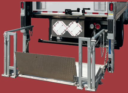
BMR-CS COLUMNLIFT
