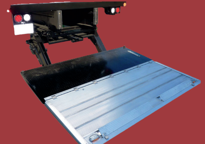
GPST SLIDELIFT
